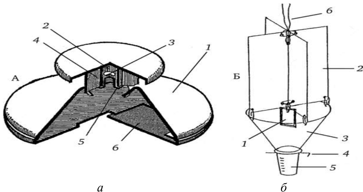
Рис. 2.3. Феромонні безклесєві пастки різних конструкцій:
