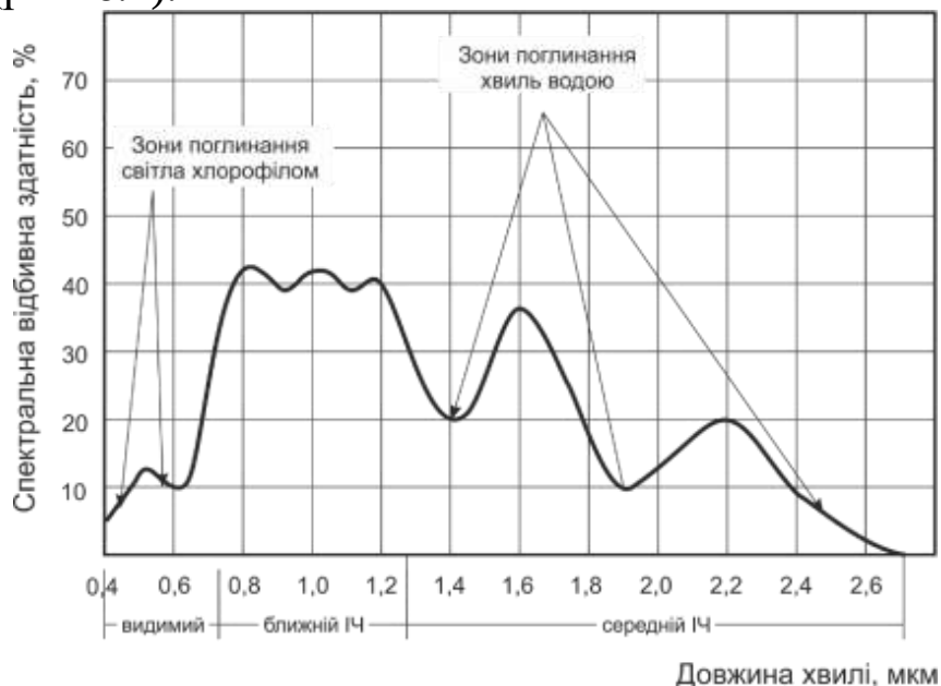
Рис. 6.1. Крива спектральної відбивної здатності зеленої рослинності
