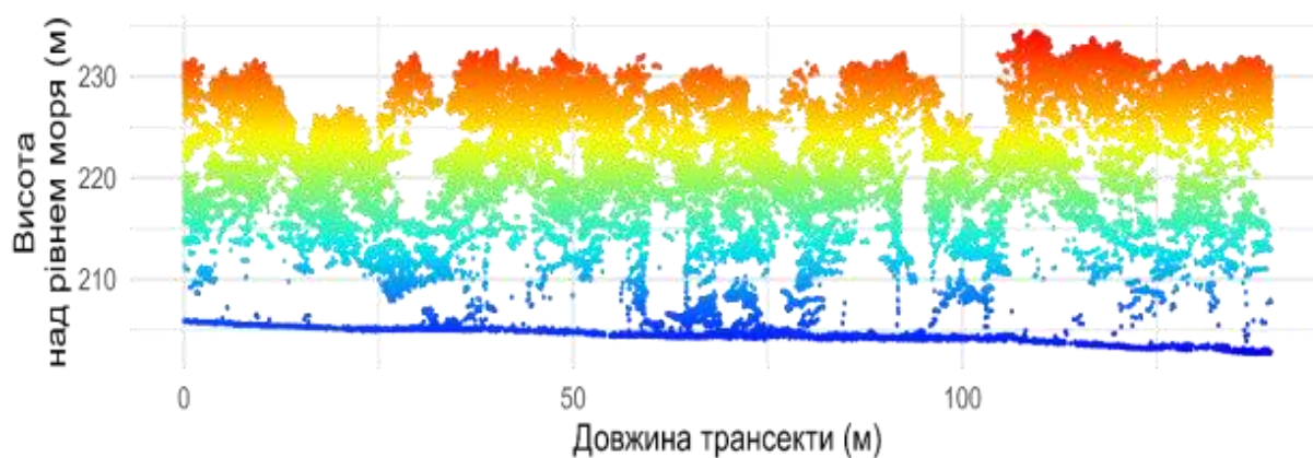
Рис. 6.3. Вертикальний профіль деревостану вздовж трансекти завширшки 5 м, одержаний за даними лазерного сканування
