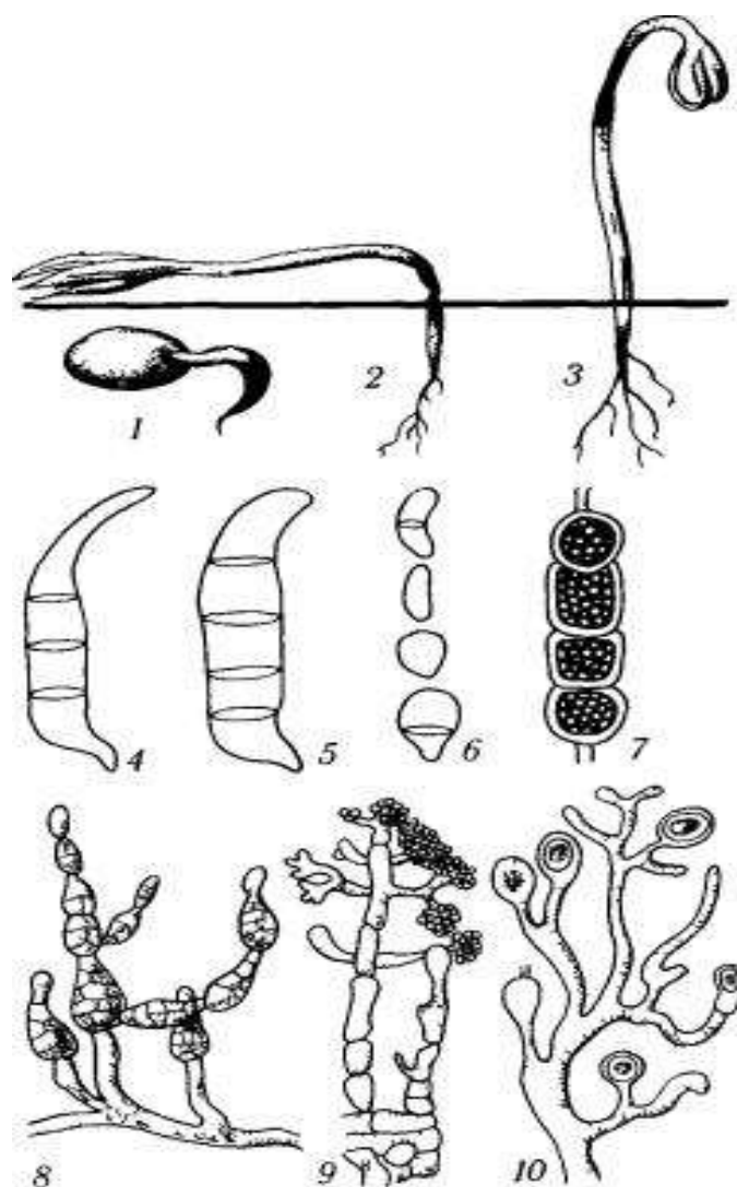
Рис. 2.6. Полягання і спороношення збудників: 1 – уражений проросток; 2 – ураження кореневої шийки сіянця хвойних; 3 – уражене підсім'ядольне коліно сіянця листяних; 4–7 – рід Fusarium (4–5 – макроконідії, 6 – мікроконідії, 7 – хламідоспори); 8 – рід Alternaria ; 9 – рід Botrytis ; 10 – рід Pythium
