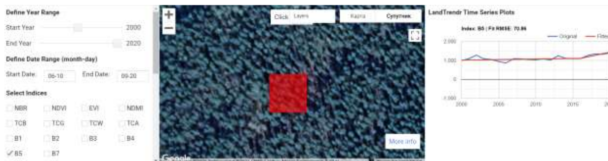
Рис. 6.4. Демонстрація алгоритму LandTrendr для ділянки соснового деревостану, пошкодженої верхівковим короїдом
